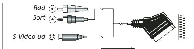
Figur 6 SCART/S-Video Adaptor til afspilning; signalretning Phono > SCART
