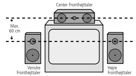
A) Fronthøjtaler installation med billedrørs-TV, fladskærm eller bagprojektion.
