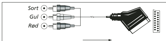
Figur 3 Phono/SCART til afspilning; signalretning Phono > SCART
