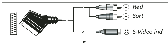
Figur 4 SCART/S-Video Adaptor til afspilning; signalretning SCART > Phono
